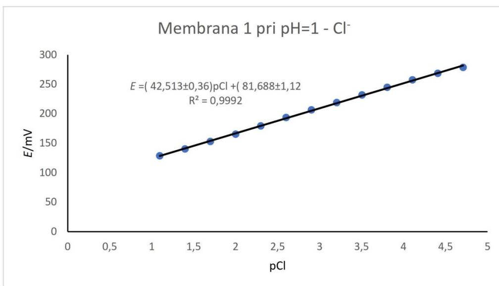
Slika 14. Prikaz testiranja odziva elektrode na \text{Cl}^- ione
