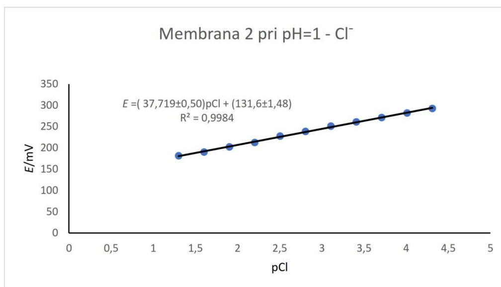
Slika 16. Prikaz testiranja odziva elektrode na \text{Cl}^- ione
