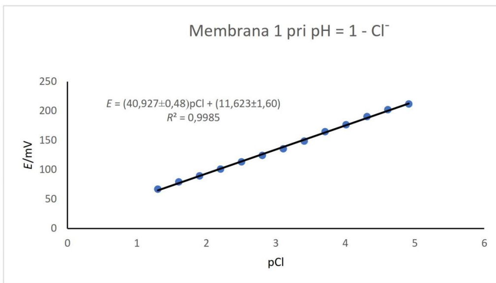
Slika 23. Prikaz testiranja odziva elektrode na \text{Cl}^- ione
