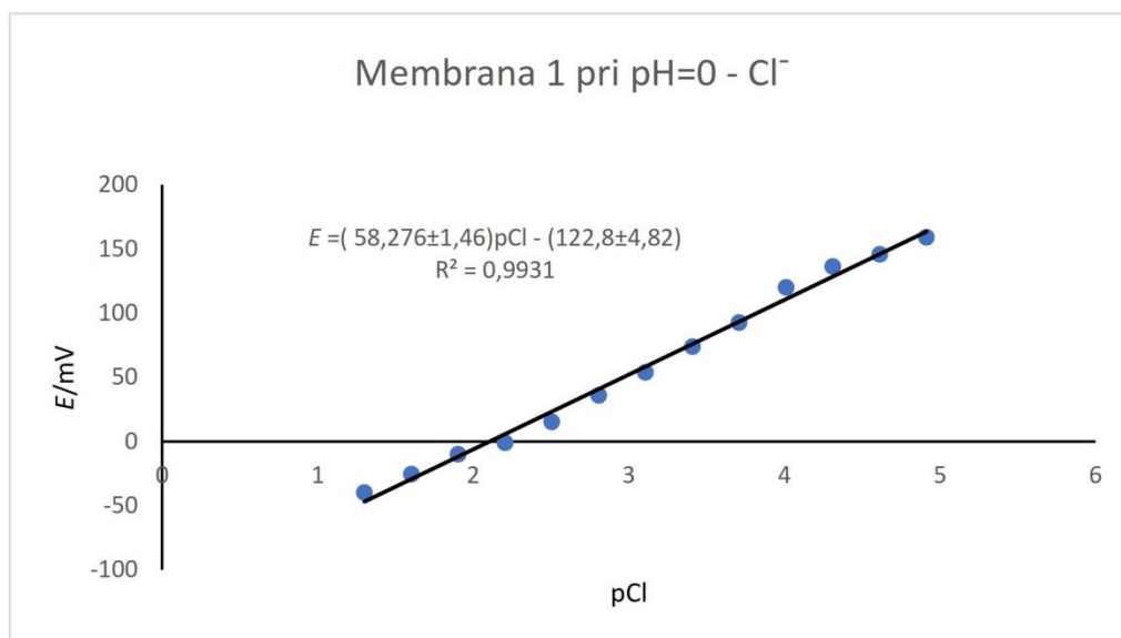
Slika 21. Prikaz testiranja odziva elektrode na \text{Cl}^- ione
