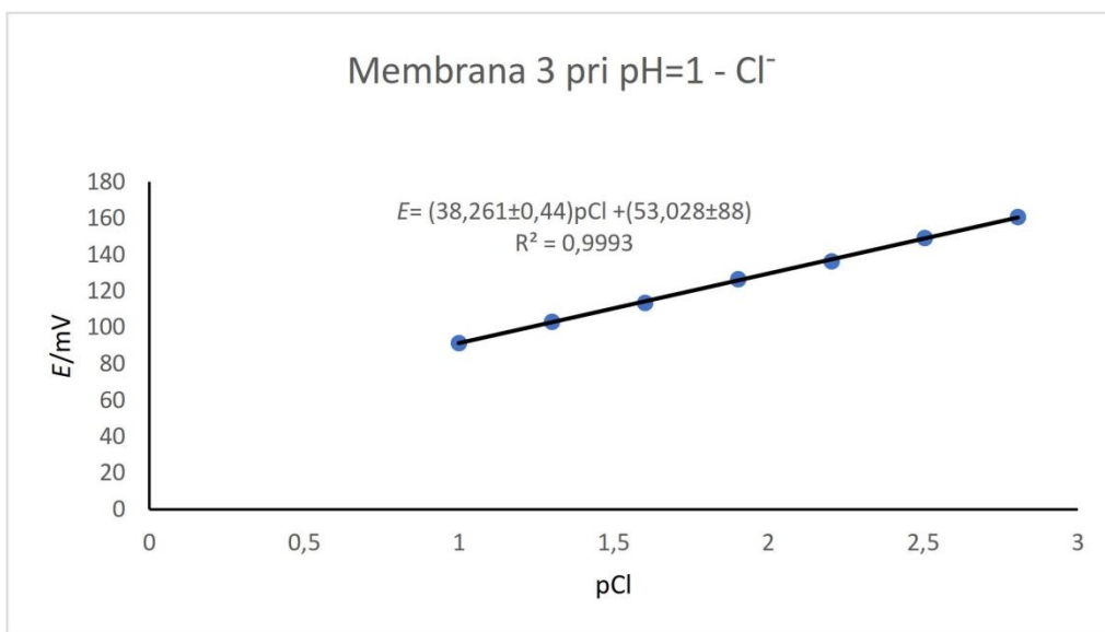
Slika 29. Prikaz testiranja odziva elektrode na \text{Cl}^- ione
