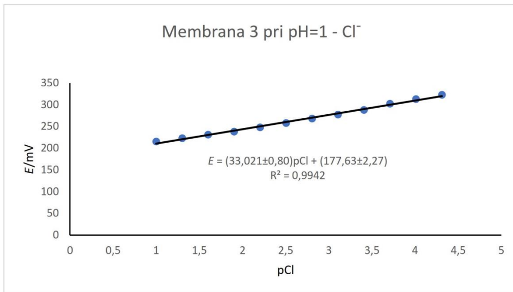
Slika 26. Prikaz testiranja odziva elektrode na \text{Cl}^- ione
