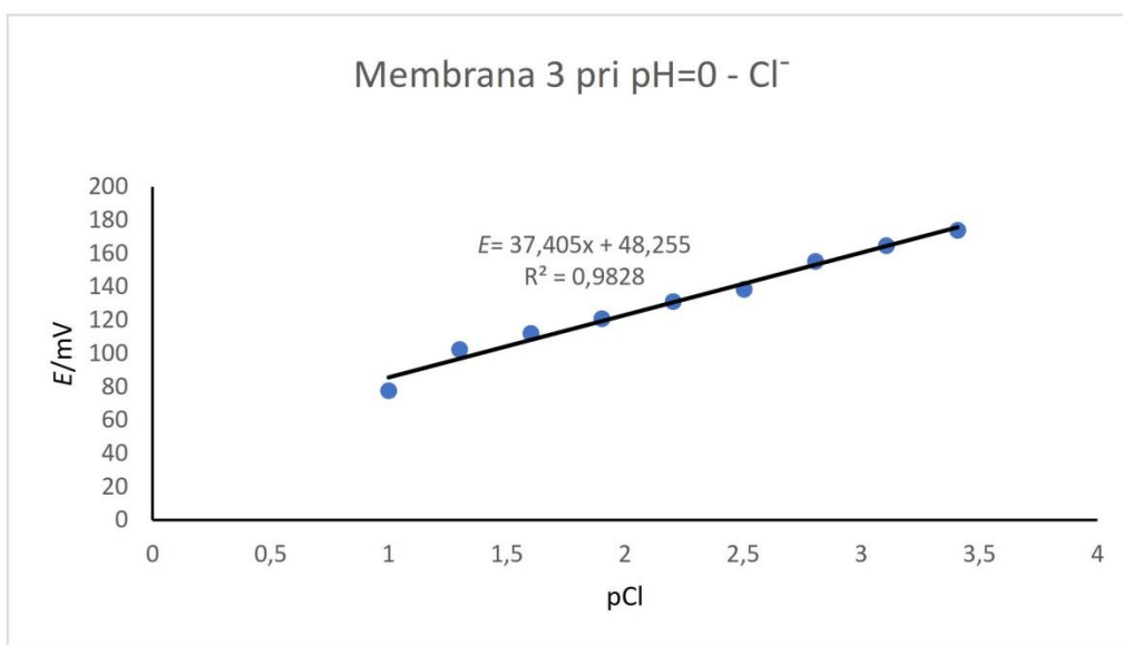
Slika 28. Prikaz testiranja odziva elektrode na \text{Cl}^- ione
