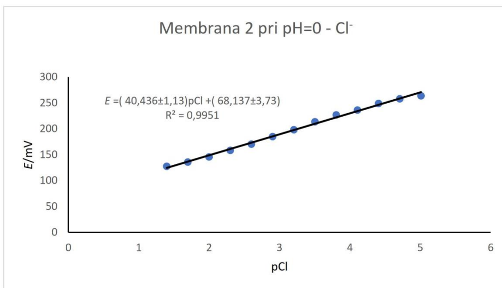
Slika 15. Prikaz testiranja odziva elektrode na \text{Cl}^- ione
