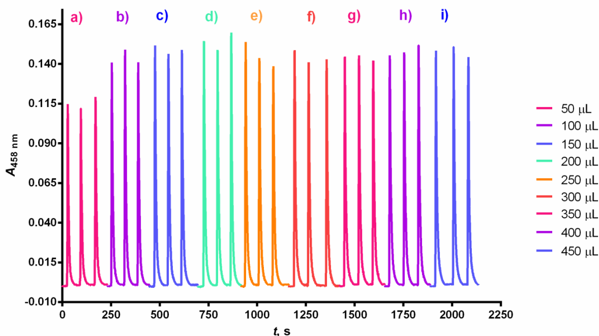
Slika 4.4. Siagram optimizacije volumena injektiranja reagensa. Eksperimentalni uvjeti: c(\text{cys}) = 4,0 \times 10^{-5} \text{ mol L}^{-1} ; c([\text{Cu}(\text{Nc})_2]^{2+}) = 1,0 \times 10^{-3} \text{ mol L}^{-1} ; \text{pH} = 3 ; protočna kiveta volumena 80 \mu\text{L} ; petlja zadržavanja od 1000 \mu\text{L} ; reakcijska petlja duljine 70 cm; volumen injektiranja cisteina = 200 \mu\text{L} ; volumen osnovne otopine = 3000 \mu\text{L} ; valna duljina pri kojoj je spektrofotometrijski bilježen signal iznosi \lambda = 458 \text{ nm} , brzina protoka = 3000 \mu\text{L min}^{-1} ; volumen injektiranja [\text{Cu}(\text{Nc})_2]^{2+} : a) = 50 \mu\text{L} , b) = 100 \mu\text{L} , c) = 150 \mu\text{L} , d) = 200 \mu\text{L} , e) = 250 \mu\text{L} , f) = 300 \mu\text{L} , g) = 350 \mu\text{L} , h) = 400 \mu\text{L} , i) = 450 \mu\text{L} .
