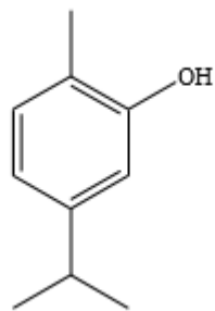
Karvakrol
