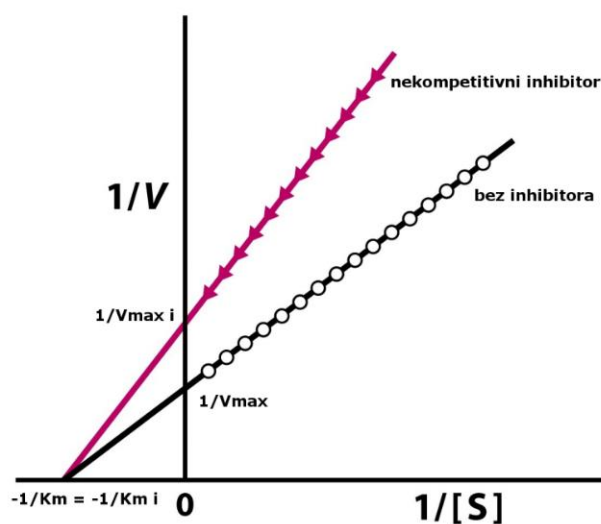
Slika 1.17. Lineweaver-Burk prikaz nekompetitivne inhibicije.
