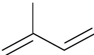
Slika 1.27. Struktura izoprena.
