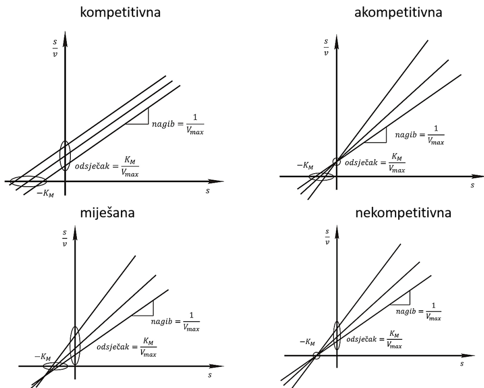
Slika 1.21. Hanes-Woolf prikaz različitih vrsta inhibicija.
