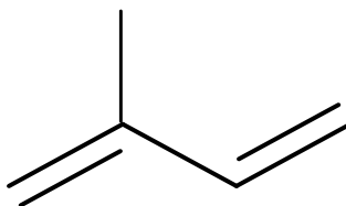
Slika 1.27. Struktura izoprena.
