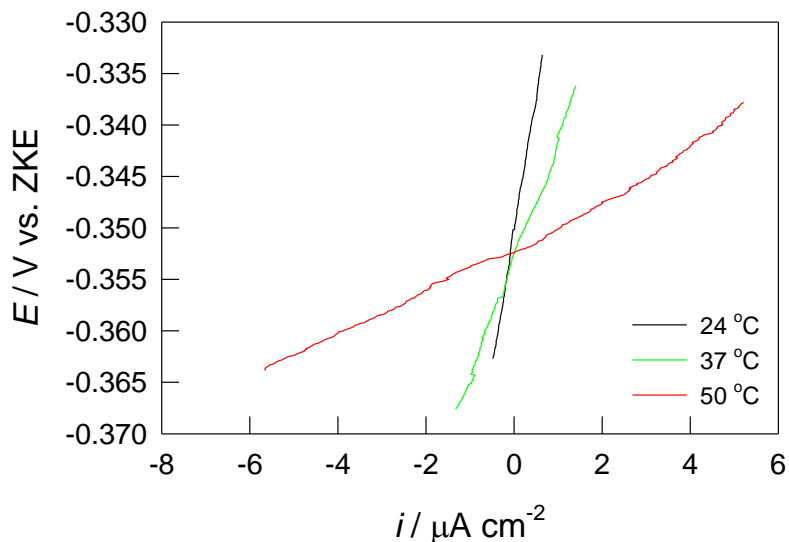
Slika 23. Linearni dijelovi polarizacijskih krivulja dobiveni metodom linearne polarizacije za CuAlNi leguru u 0,9 % NaCl otopini pri pH = 7,4 i različitim temperaturama elektrolita
