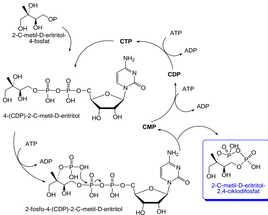
Slika 17. Nastanak 2-C-metil-D-eritritol-2,4-ciklodifosfata
