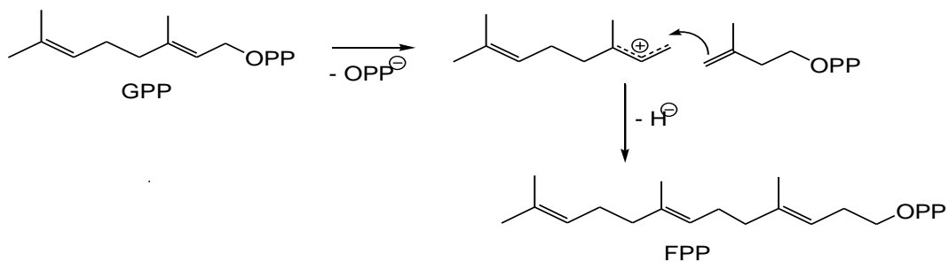
Slika 11. Nastanak farnezil-pirofosfata
