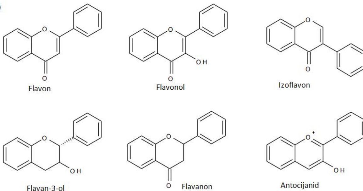
Slika 13. Osnovna kemijska struktura flavonoida (A) i opće strukture najvažnijih podklasa flavonoida (B)
