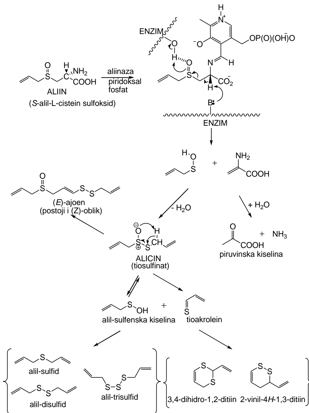
Slika 1.8. Aliinazom katalizirana konverzija aliina (S-aliil-L-cistein-sulfoksid) u alicin (tiosulfinat) i ostale isparljive organosumporne spojeve 3
