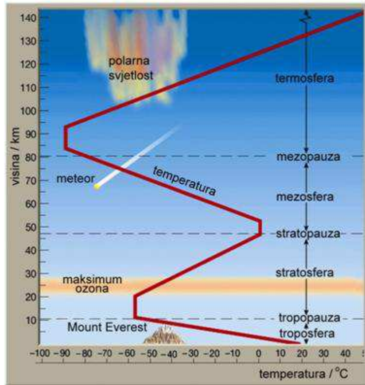
Slika 1.1. Slojevi atmosfere. 8
