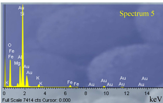
Slika 2.3. SEM snimka čestica tla onečišćenog živom i pripadajući EDS spektri
