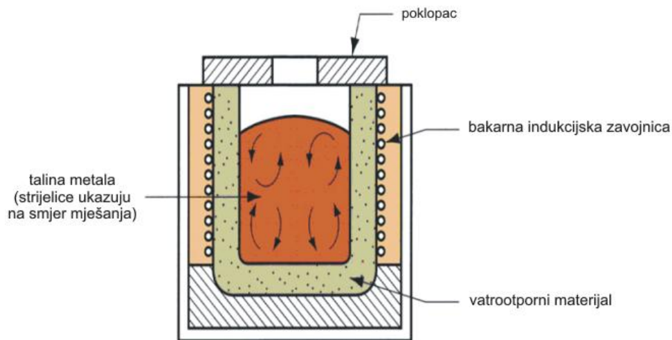
Slika 11. Shematski prikaz indukcijskog taljenja 21
