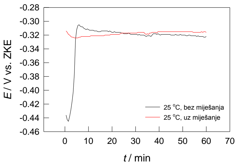
Slika 20. Vremenska ovisnost potencijala otvorenog strujnog kruga CuAlNiMn legure u 0,9 % NaCl otopini pH= 7,4, bez miješanja (-), i uz miješanje magnetskom miješalicom (-)
