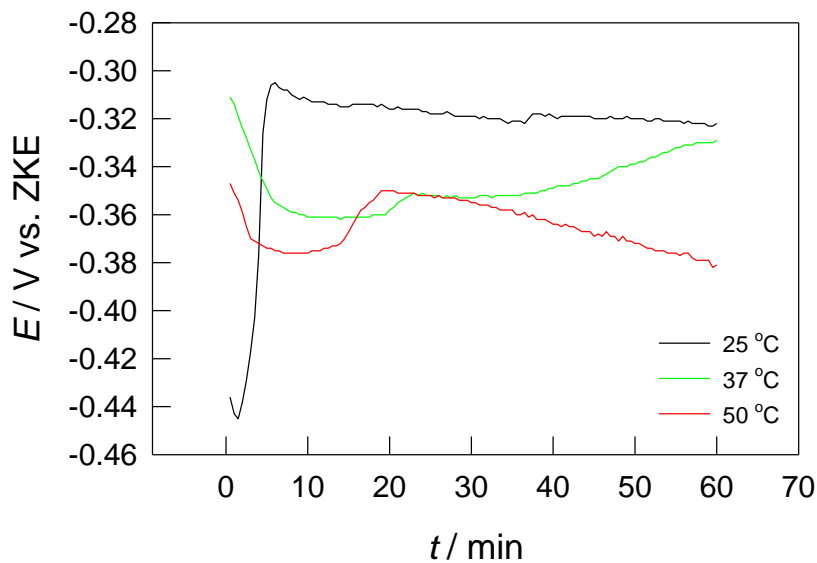
Slika 21. Vremenska ovisnost potencijala otvorenog strujnog kruga CuAlNiMn legure u 0,9 % NaCl otopini pH= 7,4, pri 25 °C (-), 37 °C (-) i 50 °C (-)
