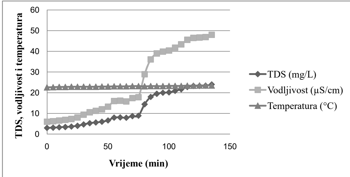
Slika 9. Ovisnost TDS-a, vodljivosti i temperature o vremenu za sintezu u ultračistoj vodi, uz dodatak vodovodne vode nakon 75 minuta sinteze, u trajanju od 135 minuta.
