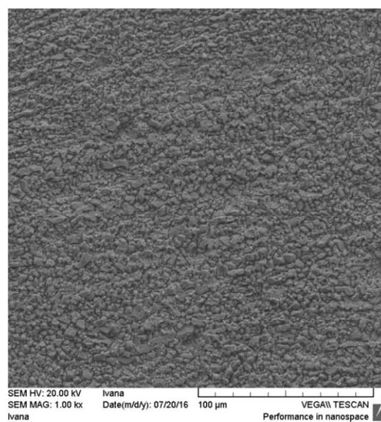
Slika 29. SEM snimke površine uzorka CuAlNi legure nakon potenciodinamičkog polarizacijskog mjerenja u 0.1 % NaCl otopini uz uvećanja od a) 46 puta; b) 100 puta; c) 500 puta i d) 1000 puta
