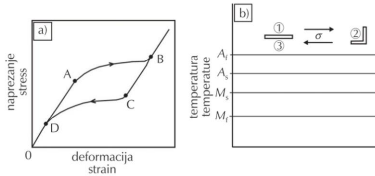
Slika 7. Dijagram naprežanje- deformacija legure s prisjetljivosti oblika a) i shematski prikaz pseudoelastičnosti b) 21
