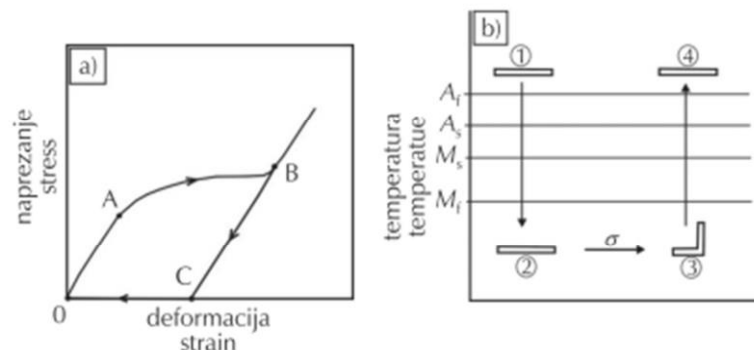
Slika 8. Dijagram naprežanja- deformacija za leguru s prisjetljivosti oblika a) i shematski prikaz
