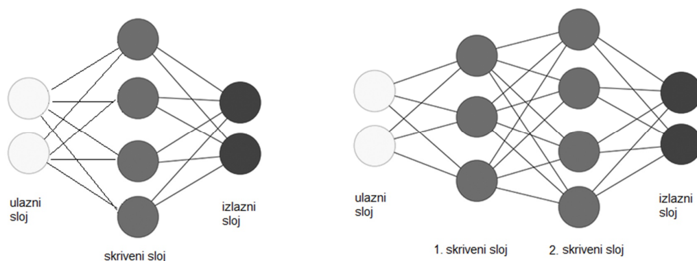
Slika.3.13. Arhitektura algoritama umjetnih neuronskih mreža 121 .
