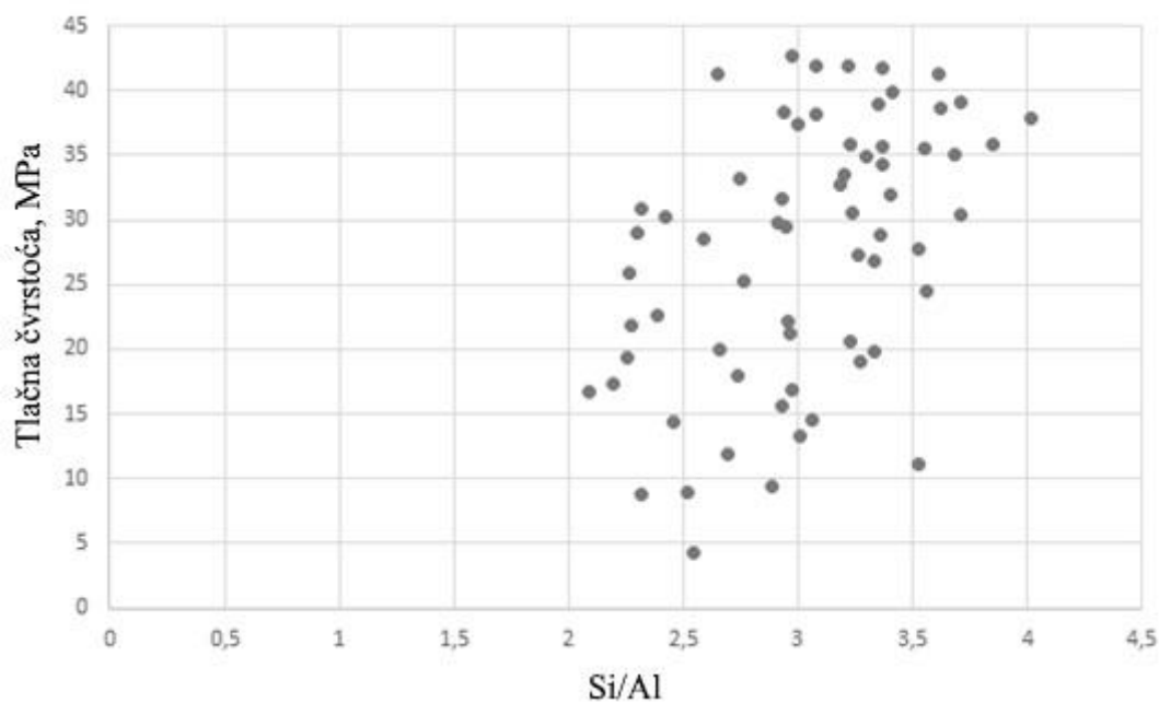
Slika 69. Ovisnost tlačne čvrstoće uzoraka serija T1 i T2 o molaranom omjeru \text{Si}/\text{Al}
