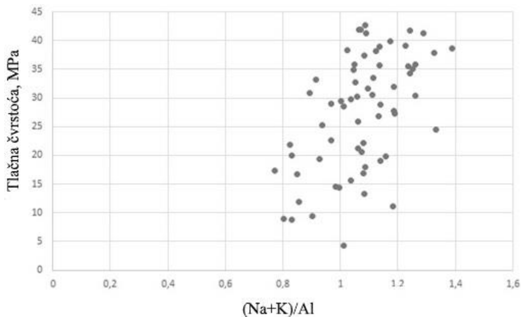
Slika 68. Ovisnost tlačne čvrstoće uzoraka serija T1 i T2 o molaranom omjeru (\text{Na}+\text{K})/\text{Al}
