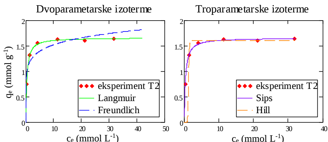
Slika 73. Procjena valjanosti izoterme s ravnotežnim eksperimentalnim podacima za uzorak T2-26 (Uvjeti: d = < 0.09 \text{ mm} , N = 200 \text{ okr min}^{-1} , t = 48 \text{ h} ).
