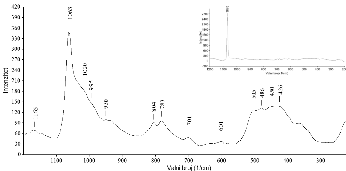
Slika 45. Ramanov spektar aktivirane mikrosilice i Ramanov spektar eflorescencije na površini aktivirane mikrosilice (manja slika)
