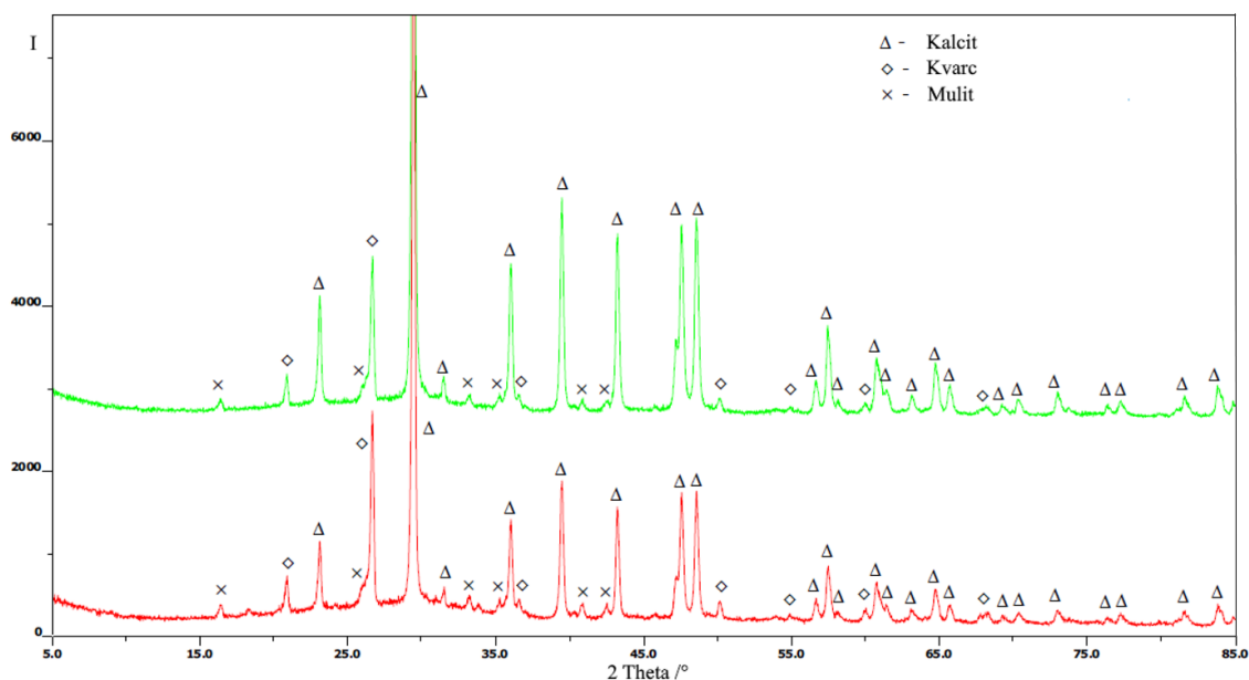
Slika 51. Rendgenski difraktrogrami uzorka T1-1 (zeleno) i T1-22 (crveno)
