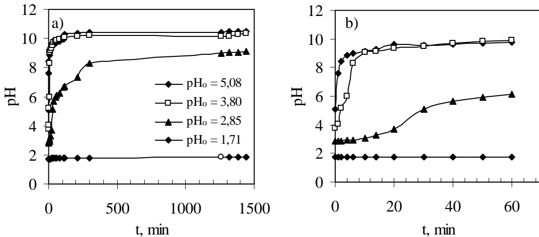
Slika 5.3. Promjena pH u sustavu FeZ - ultračista voda pri različitim početnim \text{pH}_0 vrijednostima: a) do uspostave ravnoteže i b) do 60 minuta.
