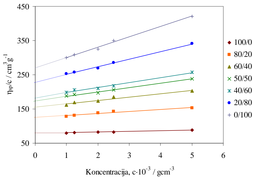
Slika 9. Ovisnost reducirane viskoznosti o koncentraciji otopine za mješavine (a) PVC/PEO1 i (b) PVC/PEO3
