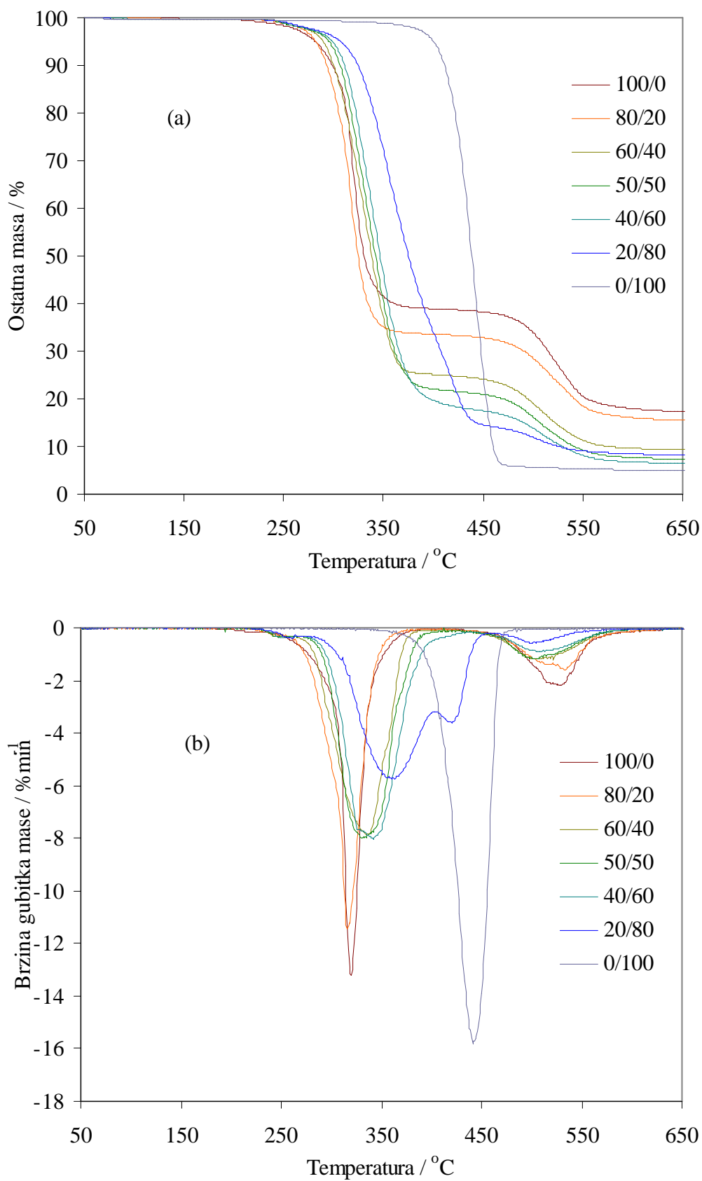
Slika 48. TG (a) i DTG (b) krivulje dinamičke TG razgradnje mješavina PVC/PEO1 različitog sastava u inerti pri brzini zagrijavanja 5 °Cmin -1
