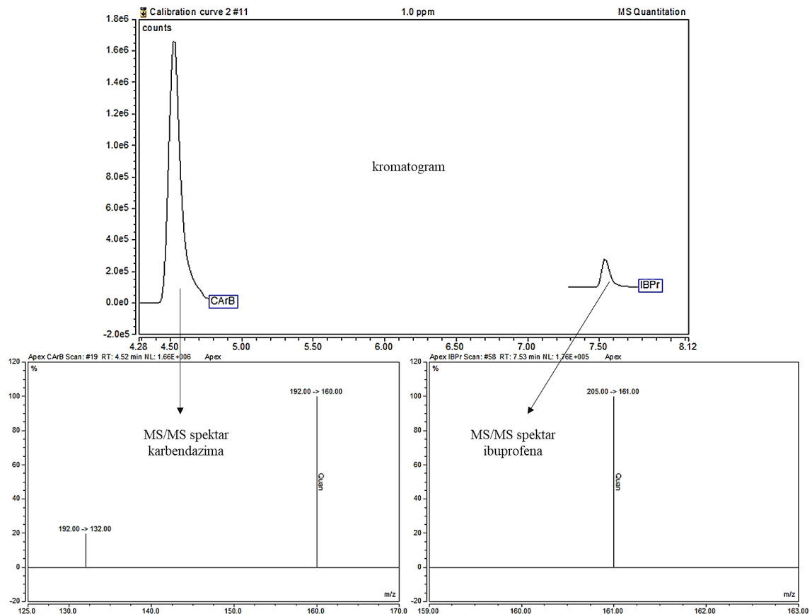
Slika 31. Kromatogram dobiven SRM načinom snimanja na spektrometru masa i spektri masa iona nastalih iz molekularnih iona ibuprofena i karbendazima.
