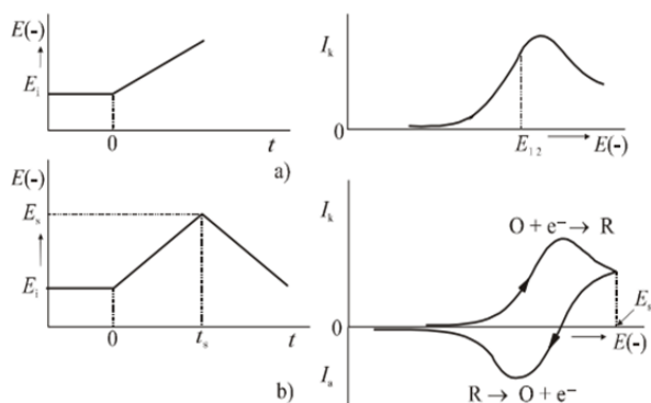
Slika 16 Signali pobude i odziva; voltametrije (a) i cikličke voltametrije (b). [24]
