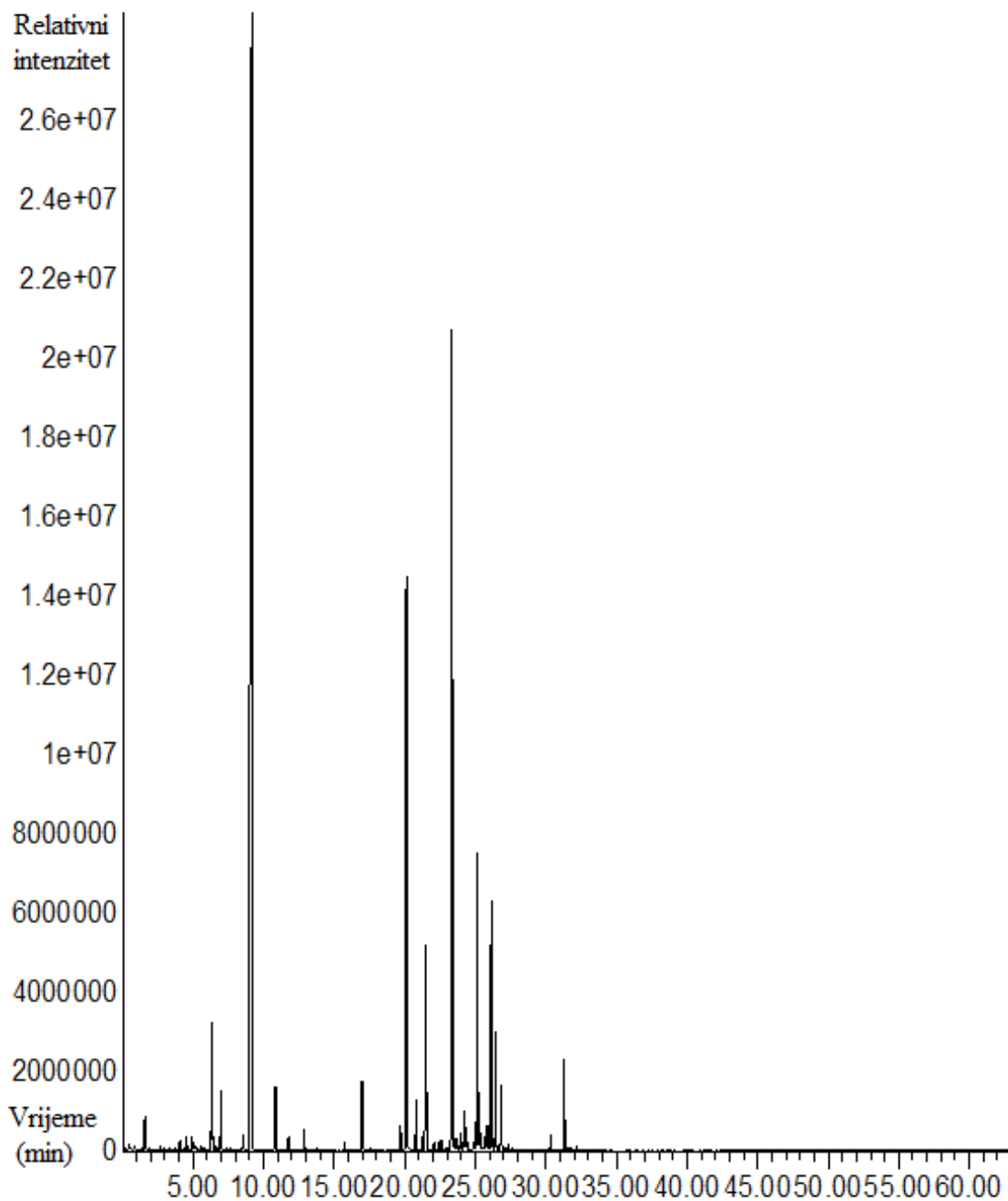
Slika 11. Kromatogram hlapljivog uzorka cvijeta bosiljka izoliranog mikroekstrakcijom vršnih para na krutoj fazi u vremenu adsorpcije od 80 minuta.
