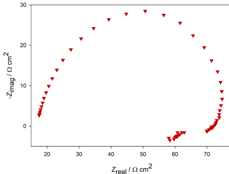
Slika 72. Nyquistov prikaz impedancijskog spektra snimljenog na elektrodi od Al 5083 legure u otopini umjetne morske vode nakon 30 dana inkubacije u biotičkom mediju.
