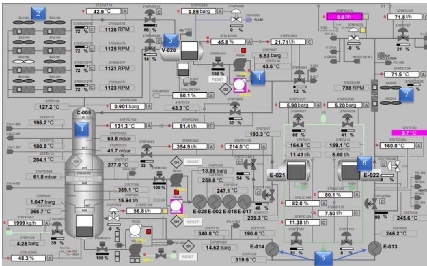
Slika 10. Shematski prikaz fracionacijske sekcije/fraktionatora:
