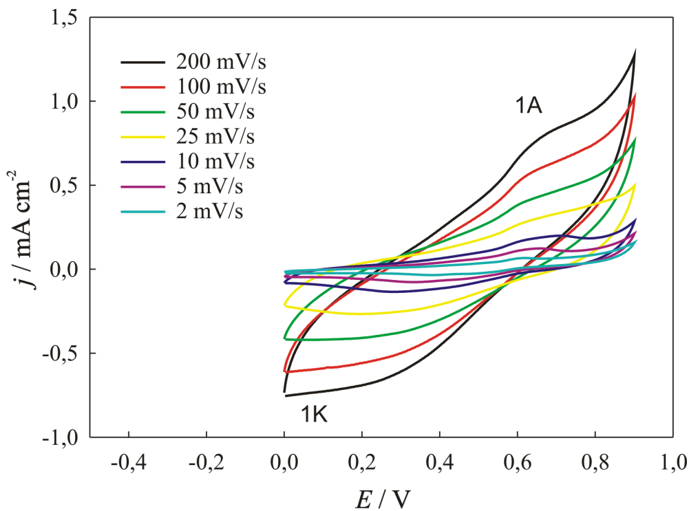
Slika 26. Ciklički voltamogrami EPG elektrode u otopini ASA u prisutnosti GK, 1 \times 10^{-4} \text{ mol dm}^{-3} – utjecaj brzine promjene potencijala, područje potencijala od 0,0 - 0,9 V.
