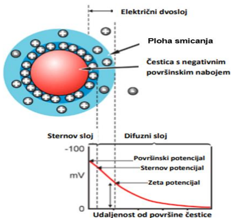
Slika 11. Shematski prikaz električnog dvosloja na površini nanočestice
