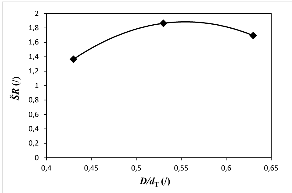
Slika 30. Utjecaj promjera SBT miješala na širinu raspodjele finalnog produkta ultrazvučne kristalizacije boraksa ( N = N_{JS} ; T_s = 30 \text{ }^\circ\text{C} ; b = 6 \text{ }^\circ\text{C h}^{-1} ; A = 20\% ; p = 20\% ).
