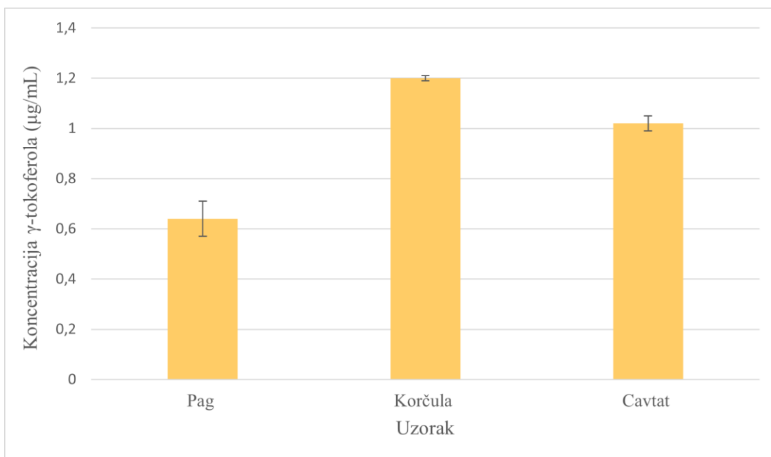
Slika 16. Grafički prikaz sadržaja \gamma -tokoferola cvijeta motra sa različitih lokaliteta
