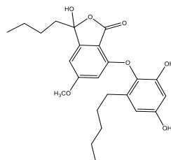
Sakisacaulon A
