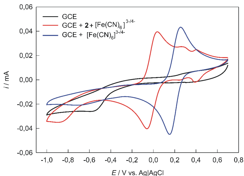
Slika 40. Ciklički voltamogrami snimljeni na GCE u 0.1 M KCl za [\text{Co}(\text{2-Br-nic})_2(\text{H}_2\text{O})_2(1,2\text{-bpeten})\times\text{DMF}]_n uz dodatak [\text{Fe}(\text{CN})_6]^{3-/4-} u otopinu ( 1\times 10^{-4} M) brzinom promjene potencijala od 10 \text{ mV s}^{-1} .
