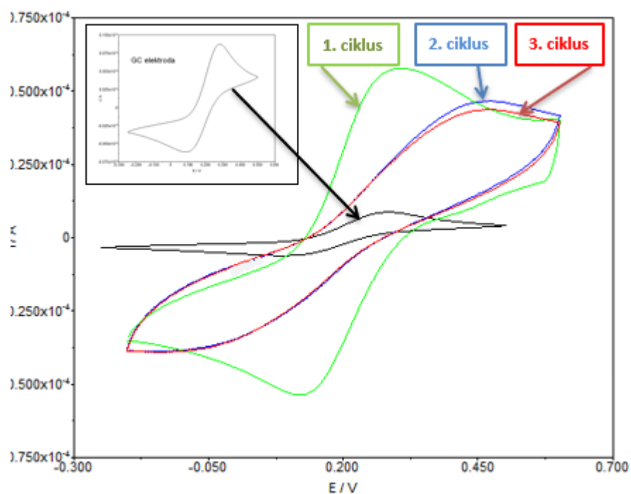
Slika 43. Ciklički voltamogram snimljen na nemodificiranoj elektrodi (crna) i Co-BPY/6-Onic modificiranoj elektrodi (2 sloja; 3 ciklusa-zeleni-plavi-crveni voltamogram) u 0,1 mol dm -3 otopini KNO 3 uz dodatak Fe 2+ /Fe 3+ .
