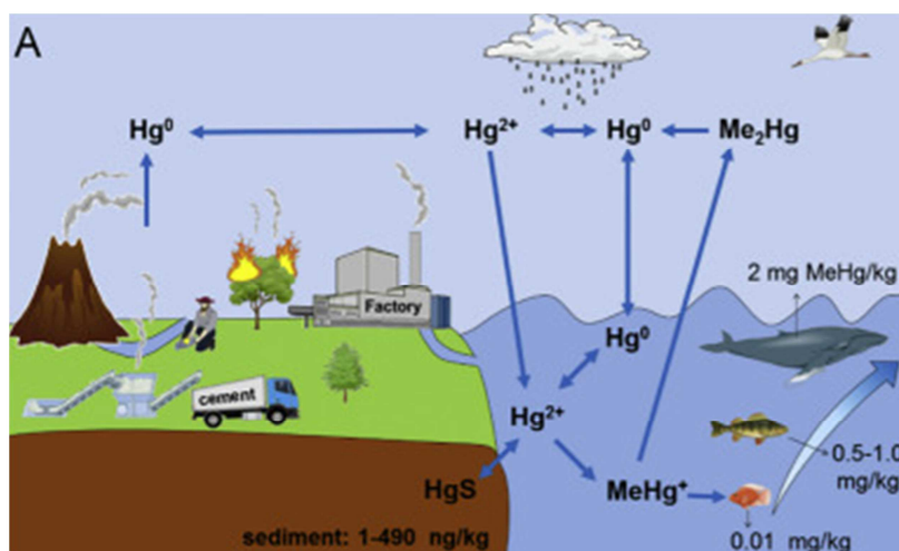
Slika 1.8. Biogeokemijski ciklus žive 18
