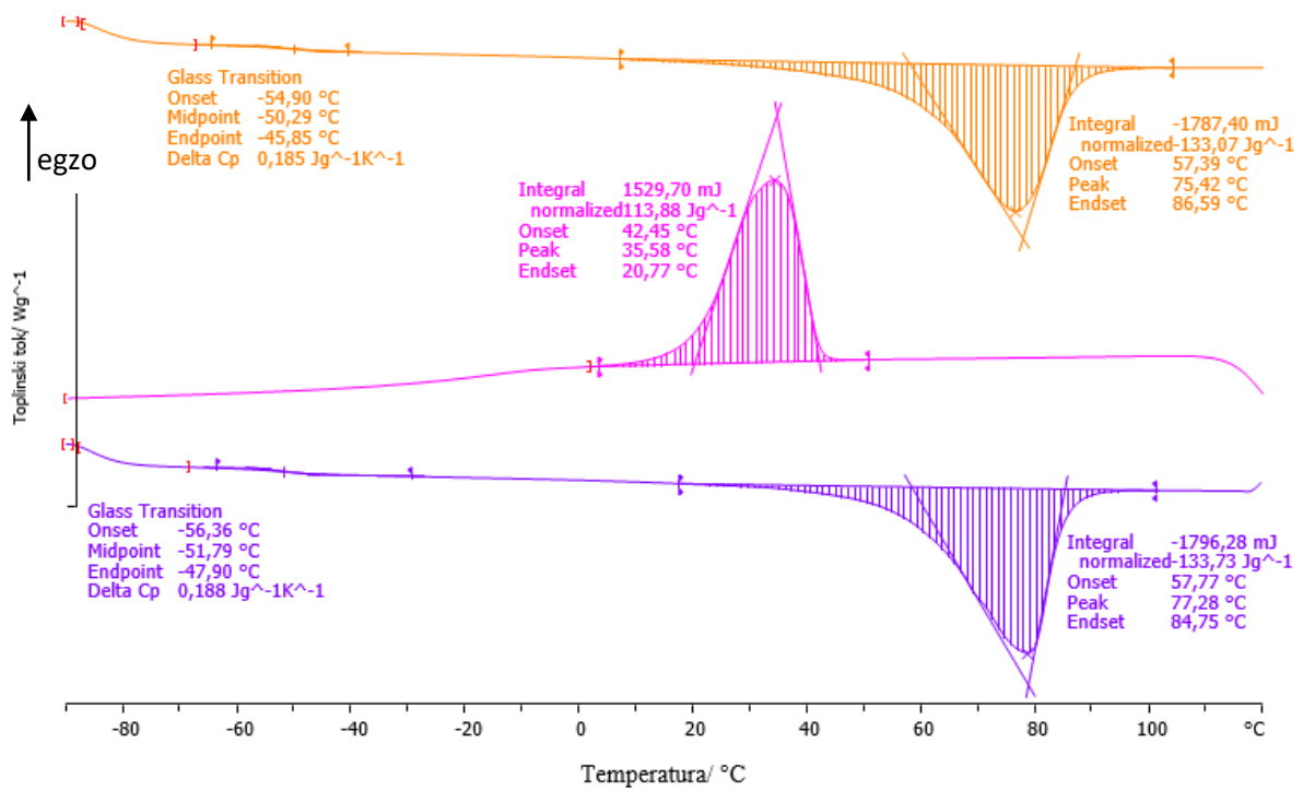
Slika 19. Normalizirane DSC krivulje uzorka PEO10
