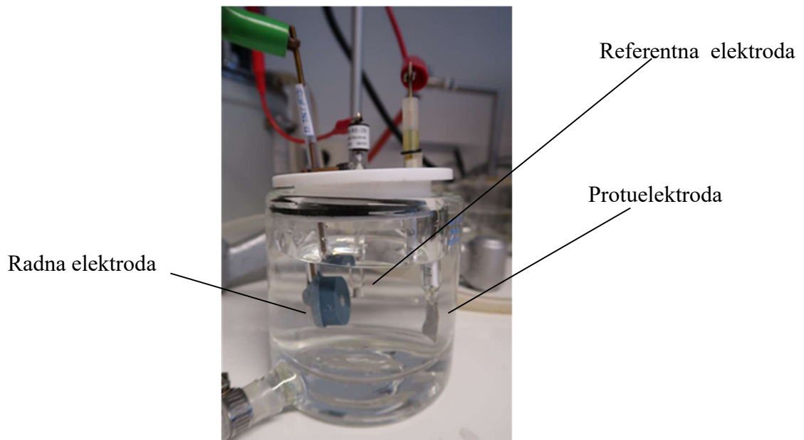
Slika 2.1. Elektrokemijski reaktor.
