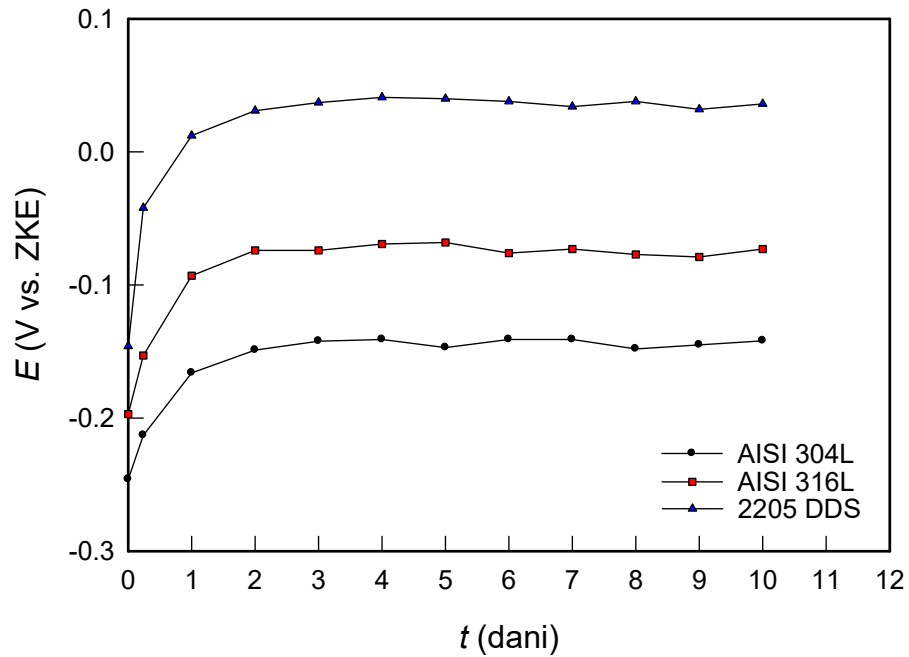
Slika 3.4. Promjena potencijala otvorenog strujnog kruga ispitivanih uzoraka u PBS otopini.
