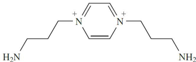
Slika 6. Ion s kojim [\text{Co(NCS-N)}_4]^{2-} daje sol crvene boje [6].
