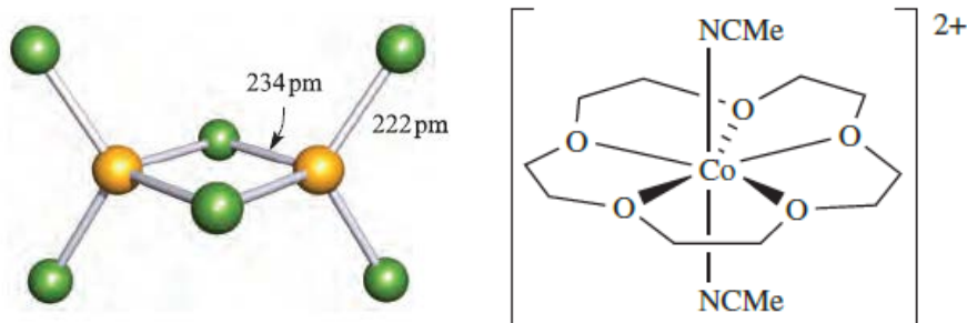
Slika 5. Struktura kompleksa [\text{Co}_2\text{Cl}_6]^{2-} (određena rentgenskom difrakcijom) i pripadajućeg kationa u soli [\text{Co(15-kruna-5)(NCMe}_2)]^{2+}[\text{Co}_2\text{Cl}_6]^{2-} (atomi kobalta su prikazani žutom, a klora zelenom bojom) [6].
