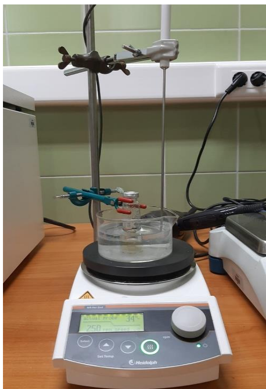
Slika 15. Aparatura za mikroekstrakciju vršnih para na krutoj fazi
