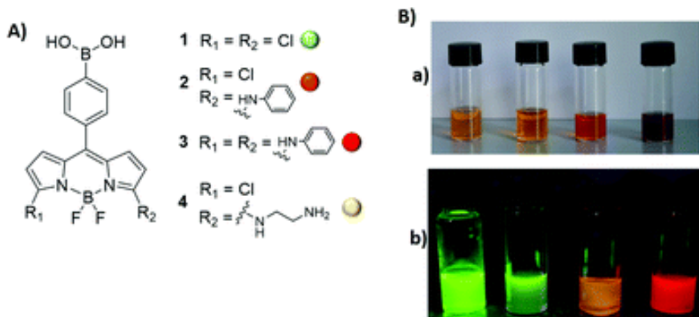
Slika 2. (A) Struktura derivata PBA-BODIPY. (B) Otopina (1,0 mg mL -1 u MeOH) derivata PBA-BODIPY (s lijeva na desno PDA-BODIPY 1, 4, 2, 3) (a) pod bijelim svjetlom i (b) pod UV-svjetlom ( \lambda_{ex} = 364 nm).
