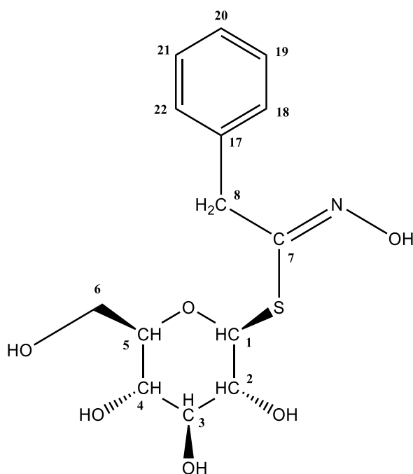
Slika 4.5.3. Struktura desulfoglukotropoepolina ( d11 ).
