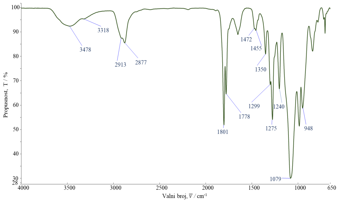
Slika 25. FT-IR spektar uzorka PEO10/LiBOB
