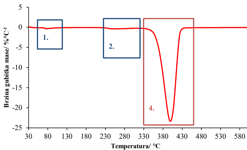
Slika 32. DTG krivulja neizotermne toplinske razgradnje 90PEO/10MgAlg
