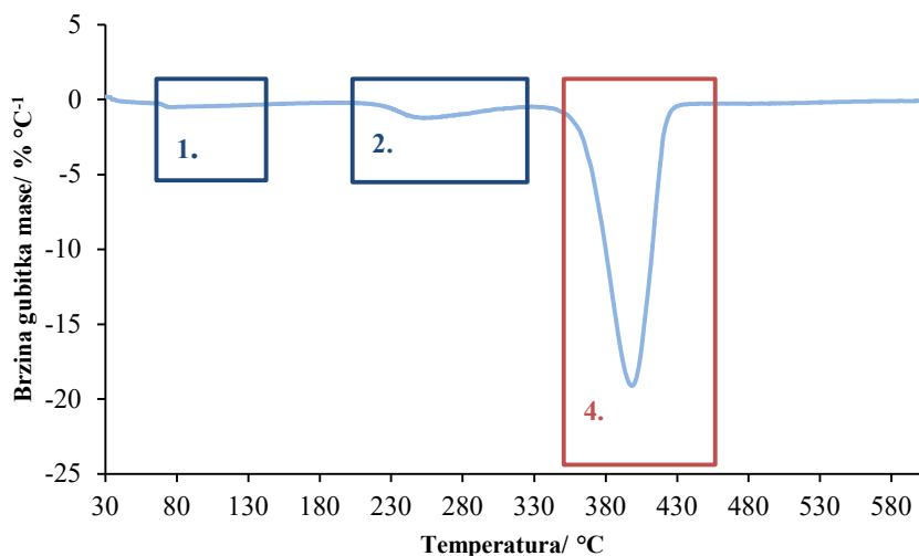
Slika 36. DTG krivulja neizotermne toplinske razgradnje 70PEO/30MgAlg
