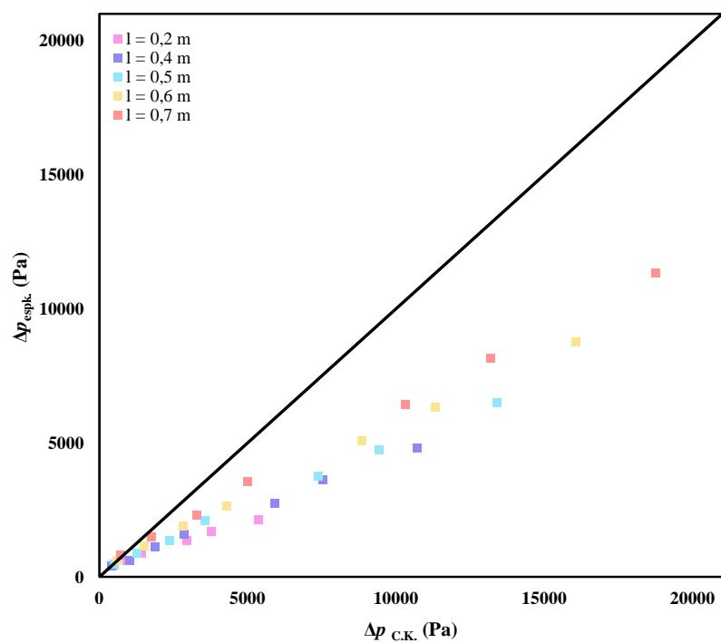
Slika 28. Usporedba eksperimentalno određenih vrijednosti pada tlaka kroz porozni sloj s vrijednostima određenim Carman-Kozenyevom i Burke-Plummerovom jednađbom ( d_{\check{c},\text{ekv.}} = 0,0065 m, \varepsilon = 0,300 ).
