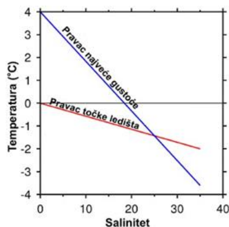
Slika 5. Ovisnost temperature leđišta o salinitetu. 17
