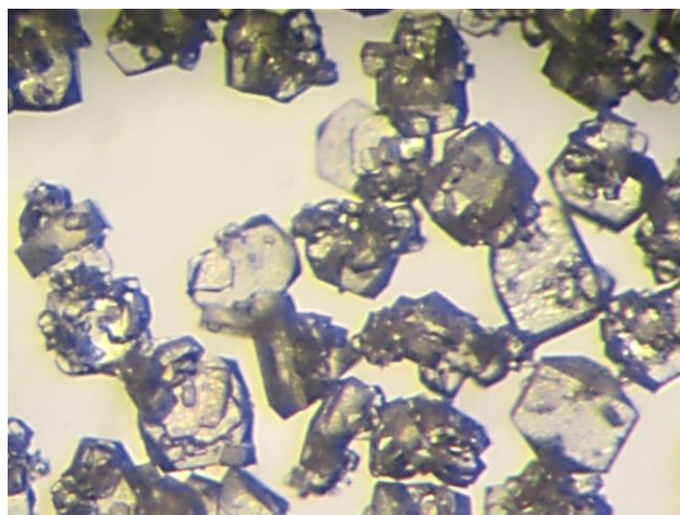
Slika 28. Kristali boraksa grube frakcije x = 275 \mu\text{m} dobiveni u sustavu bez djelovanja ultrazvuka pri D_2/d_T = 0,53 ( N = N_{JS} , T_s = 30 \text{ }^\circ\text{C} , b = 6 \text{ }^\circ\text{C}^{-1} , A = 0 \% ).
