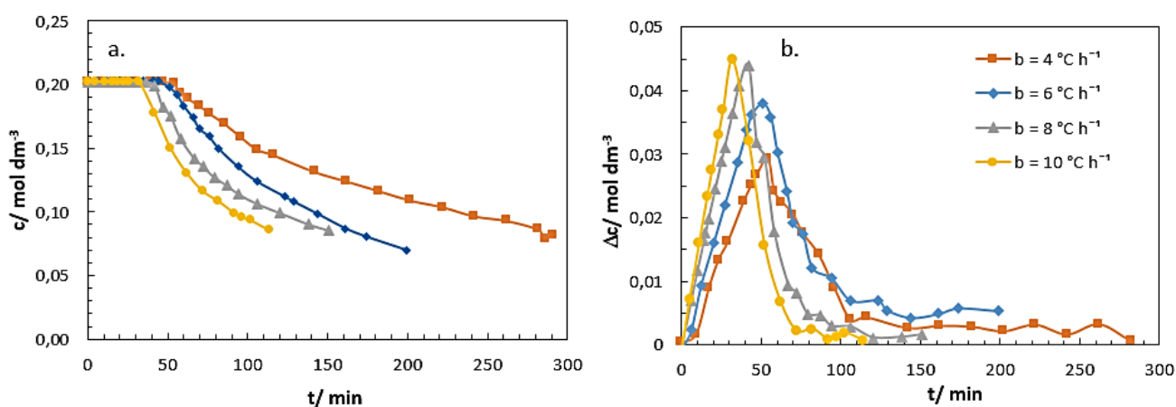
Slika 24 a) Promjena koncentracije matične otopine i b) promjena prezasićenosti tijekom procesa kristalizacije pri primjenjenim brzinama hlađenja ( A = 20 \% , T_z = 30 \text{ °C} , N_{JS} = 324 \text{ o min}^{-1} ).
