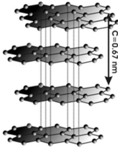
Slika 6. Građa ugljika 13
