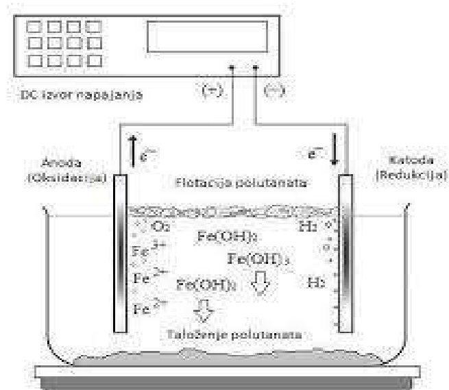
Slika 1.7. Shematski prikaz procesa elektrokoagulacije
