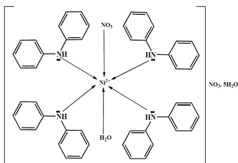
Slika 24. Prikaz oktaedarske strukture [\text{Ni}(\text{difenilamin})_4(\text{NO}_3)(\text{H}_2\text{O})(\text{NO}_3)_2 \cdot 5\text{H}_2\text{O}]^{16}
