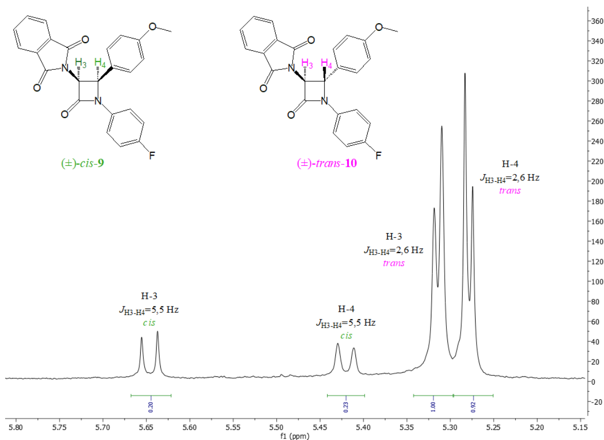
Slika 31. ^1\text{H} NMR spektar (CDCl 3 , 300 MHz) \beta -laktamskih protona H 3 i H 4 diastereoizomerne smjese (\pm) - cis - 9 i (\pm) - trans - 10
