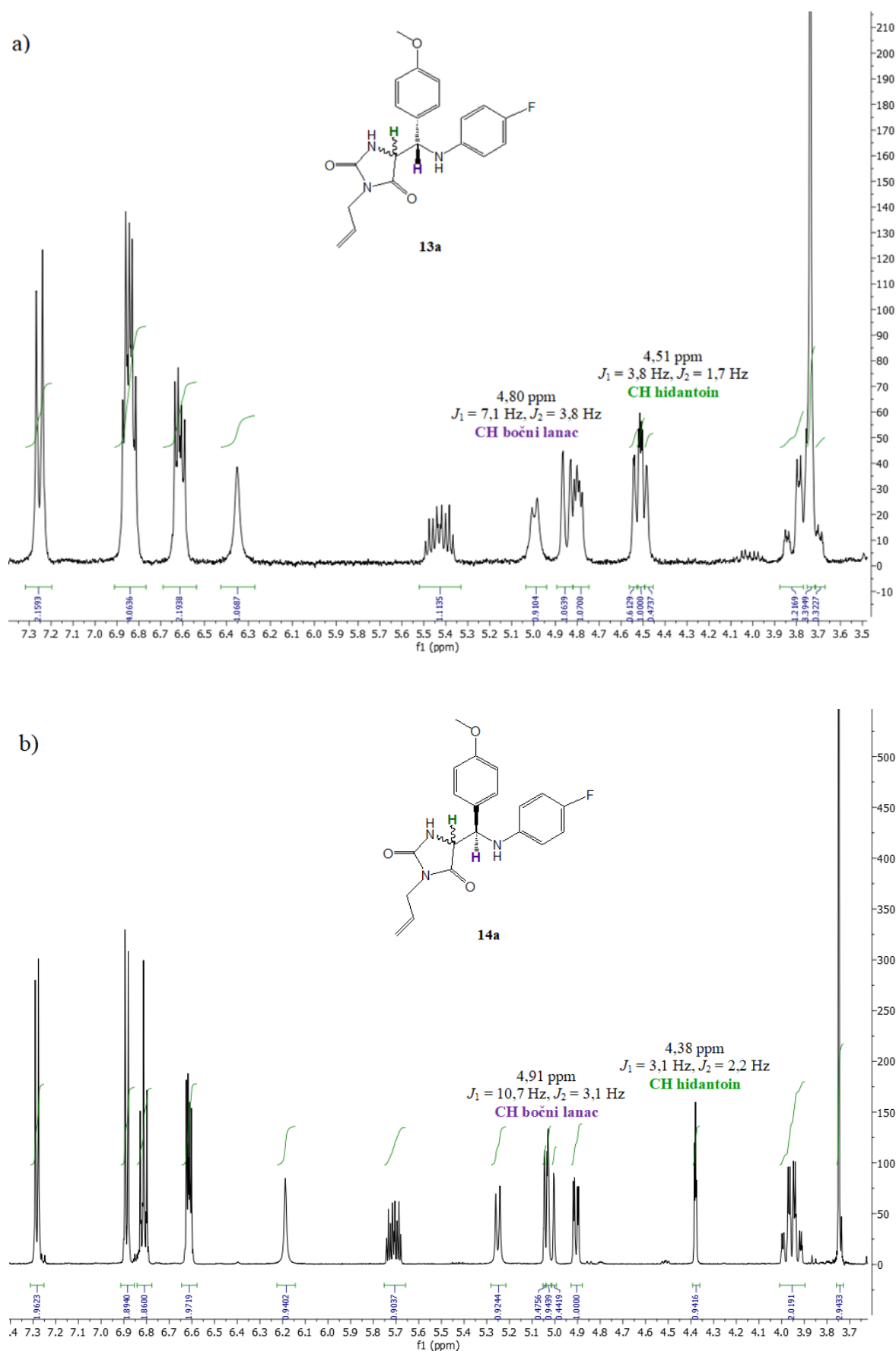
Slika 34. ^1\text{H} NMR spektari ( \text{CD}_3\text{CN} , 600 MHz) hidantoina 13a i 14a s alilnim supstituentom na N-3 položaju hidantoinskog prstena
