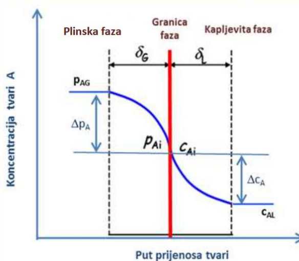
Slika 13. Dijagram teorije dvaju filmova.
