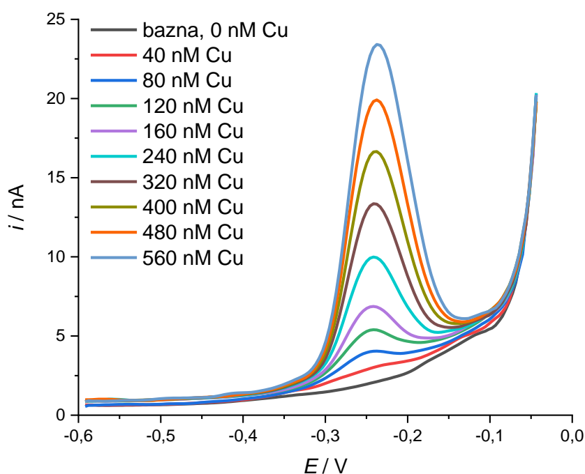
Slika 22. DPASV voltamogrami oksidacije bakra za uzorak mikrosloja mora (15_JSML), vrijeme dušiciranja 300 s, E_a = -0,6 \text{ V} , E_d = -1,4 \text{ V} , t_a = 120 \text{ s} , [\text{T-X-100}] = 1 \text{ mg/L} .
